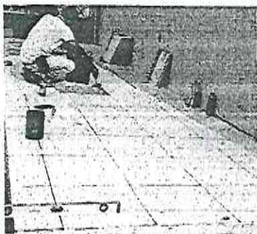
Foto 1: Instalación piso cerámico en aula.
