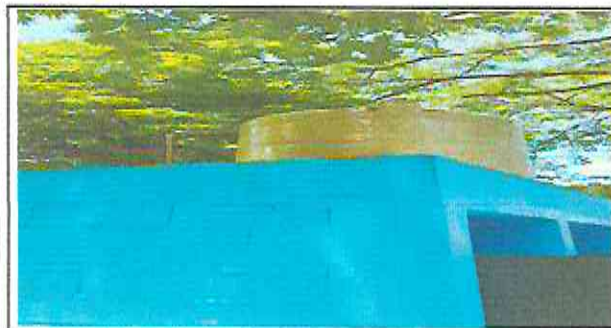
Foto 5: Sustutición de deposito de agua de 1100 litros
