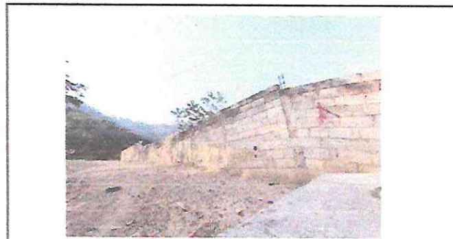
Foto 4: Reforzamiento muro perimetral
