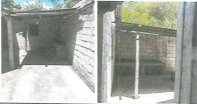
Foto 7: área de comedor, sustitución de lámina, por lámina troquelada aluzinc calibre 26 y Sustitución de estructura de soporte de madera por metal.
