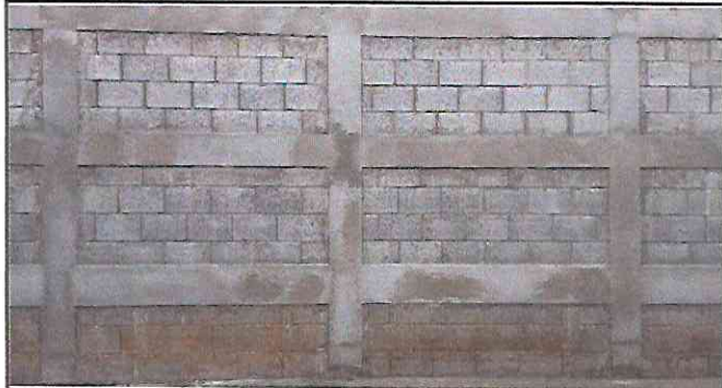
Foto 1: Sustitución cerramiento de lámina por muro de mampostería reforzada.
