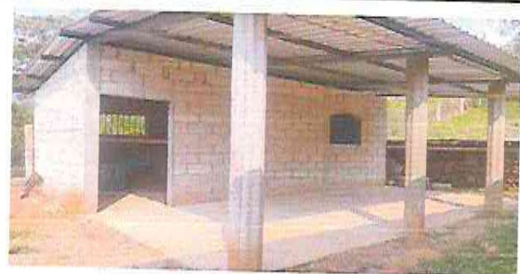
Foto 6: colocación de piso cerámico
