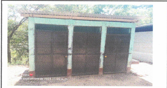
Foto 1: Mantenimiento de estructura de soporte de metal y ampliación de techo.
