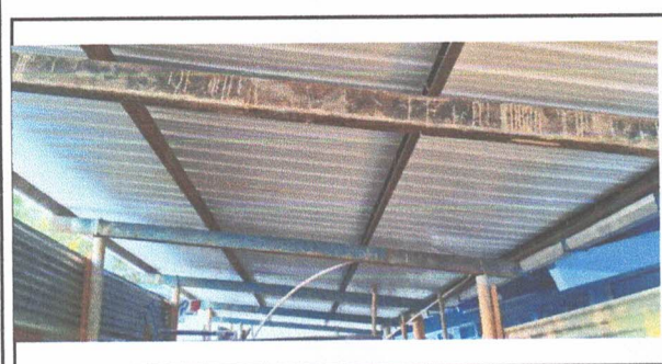
Foto 5: REPARACIÓN DE SISTEMA ELECTRICO CON LAMPARAS, CABLE, TUBERIA, CAJAS, PLAFONERAS Y LUMINARES DE 50 W.
