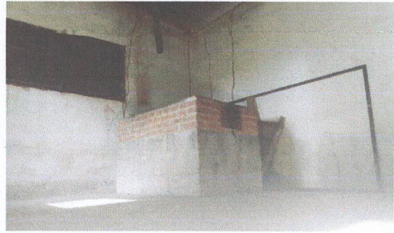
Foto 2: Sustitución de polletón, plancha y chimenea
