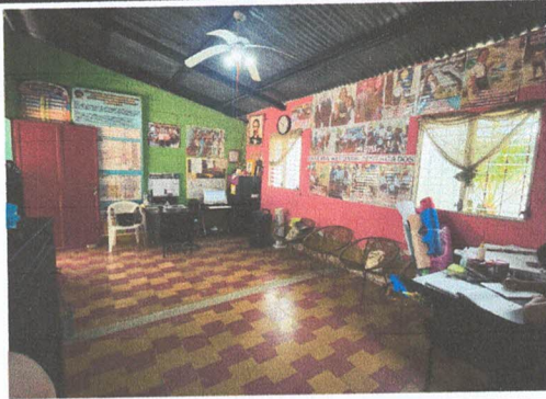
Foto1: Módulo de dirección, cambio de piso, abrir vano de 2.00x1.10mts e instalar puerta corrediza de PVC, 2.00x2.10mts y sustitución de ventanas por PVC. De 1x1 mts.
