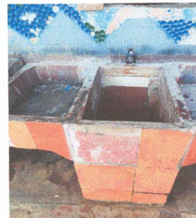
Foto 6: Sustitución e instalación de 3 pilas prefabricadas de cemento.
