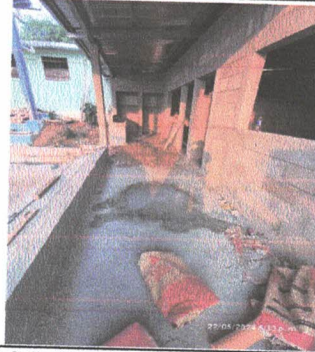
Foto 2: Corredor: Aplicación de piso torta de cemento, instalación de piso cerámico, blanqueado en muros, instalación de balcones, instalación de barandal, instalación de sistema eléctrico.
