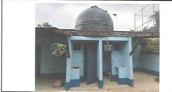
Foto 4.3 Instalacion de Tinaco existente con accesorios
