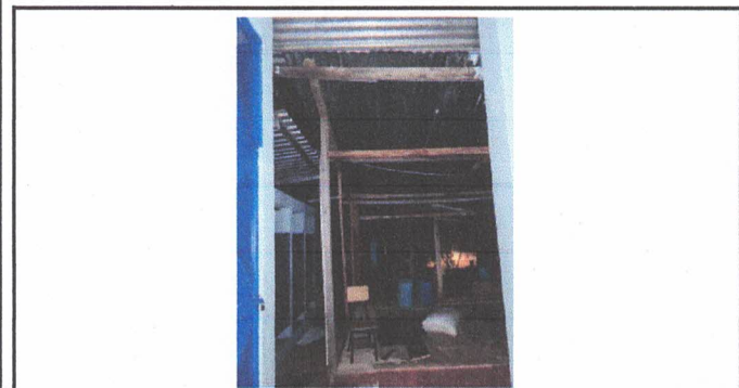
Foto 3: Reparación de Techo en Area de Pila se cambiará cubierta provisional a Cubierta de Techo con costanera y Lamina Aluzinc Troquelada Calibre 26 Legitima.
