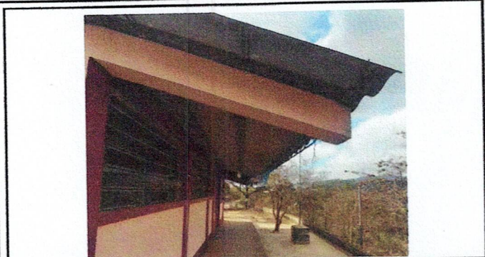
Foto 1: Reparación de 2 Aulas y Corredor de Escuela de Parvulos. Cambio de Lámina de Asbesto cemento a Lámina Troquelada de Aluzinc Calibre 26 Legítimo.
