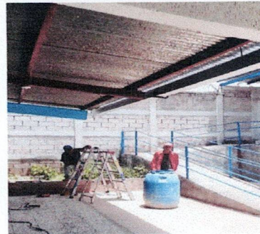
Foto 4: Sustitución de bajada de agua pluvial de metal por tubo PVC 3"
