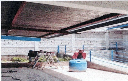
Foto 5: Sustitución de bajada de agua pluvial de metal por tubo PVC 3"
