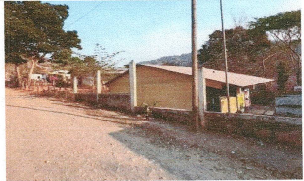
Foto 2: Reparación de Muro Perimetral: En la parte frontal se trabajará Malla en marcos para la parte superior, se resanara el muro frontal, se reparará cuneta o acceso peatonal, reparación de gradas internas y se pintará con pintura latex.
