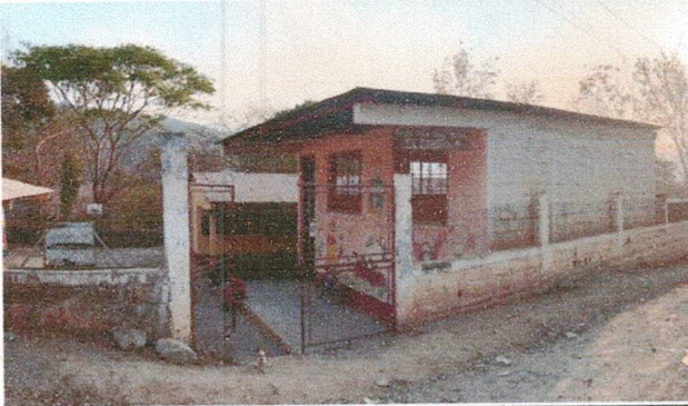
Foto 1: Reparación de Muro Perimetral: En la parte frontal se trabajará Malla en marcos para la parte superior, se resanara el muro frontal, se reparará cuneta o acceso peatonal, reparación de gradas internas y se pintará con pintura latex.
