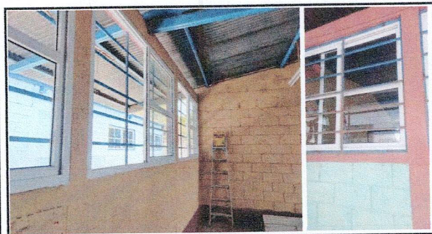
Foto 3: Instalación de ventanería de PVC y se deja la estructura de las ventanas de metal existentes como balcones.
