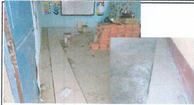
Foto 1: Instalacion de piso ceramico en aulas.
