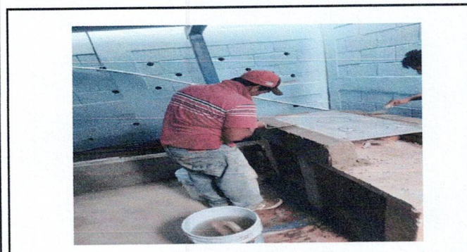
Foto 9: Construcción de Estufa Rural Completa
