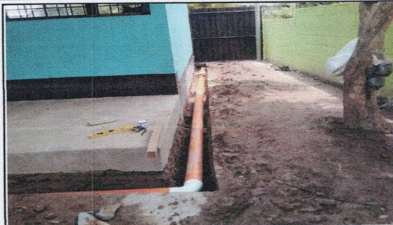
Foto 8: INSTALACIÓN DE TUBERIA PVC EN LÍNEA PRINCIPAL DE AGUA PLUVIAL
