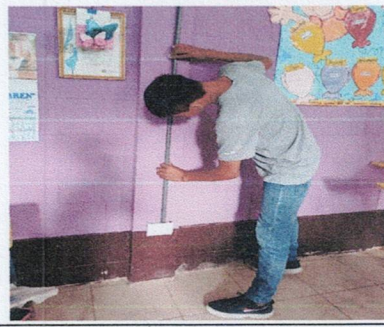
Foto 4: SUSTITUCION DE UNIDAD DE FUERZA (CAJA, TOMACORRIENTE, ALAMBRADO Y DUCTO)
