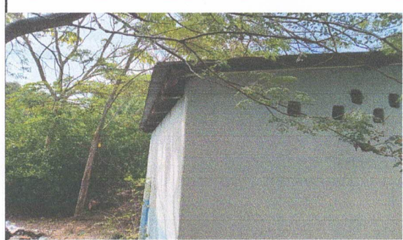
Foto 4: DEMOLICIÓN E INSTALACIÓN DE VENTANA DE METAL.
