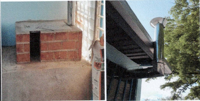
Foto 1 Instalación de estufa rural completa
