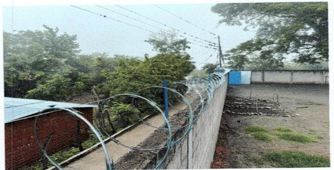
Foto 6 Protección de muro perimetral con Razor Ribbon
