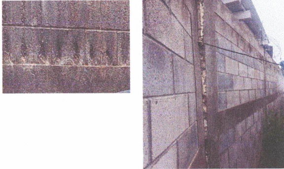
Foto1: AULAS: Instalación de Muro de Block
