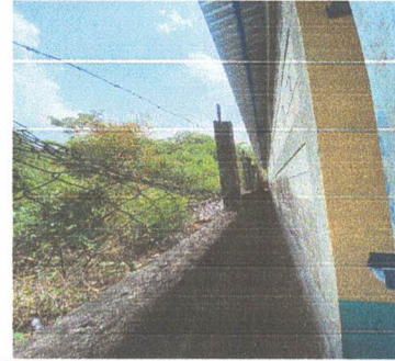
FOTO 2: REPARACIÓN DE MURO PERIMETRAL DE BLOCK (SUSTITUCIÓN DE MAYA POR BLOCK)
