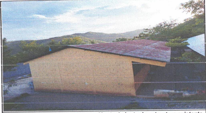
Foto2: Retiro de lámina existente, Mantenimiento de estructura existente (limpieza, lijado y pintura anticorrosiva), instalación de lámina troquelada aluzinc cal. 26 y mantenimiento de puertas.
