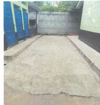
Foto 4: SUSTITUCIÓN DE PLANCA DE CONCRETO EN PATIO ✓
