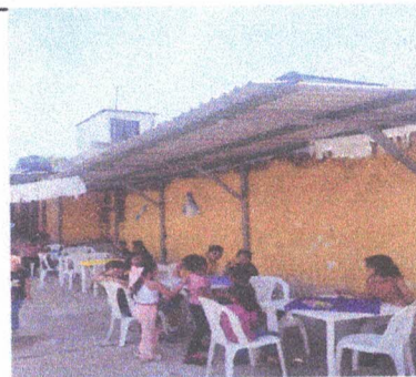
Foto 6: INSTALACION DE LAMINA TROQUELADA ALUZINC CAL 26
