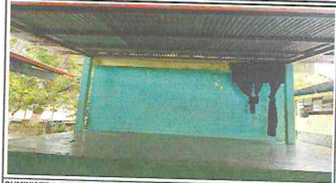
SUMINISTRO E INSTALACION DE 142 M 2 DE ESTRUCTURA DE METAL Y 142 M 2 DE LAMINA TROQUELADA ALUZINC CALIBRE 26 EN AREA DE ESCENARIO Y AREA CONTINUA A CUARTO GRADO.
