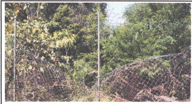
Reparación de muro perimetral de block hg y malla galvanizada, soleras intermedias y columnas
