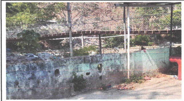
Reparación de muro perimetral de block con tubo hg y malla galvanizada, soleras intermedias y columnas
