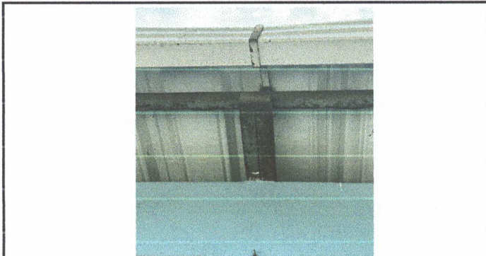
Foto 3: Sustitución de estructura de soporte de metal (Costanera) por estructura de similar consistencia
