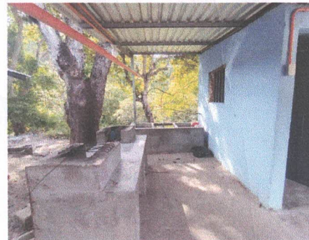
INSTALACIÓN PARA CERRAMIENTO CON BLOCK Y MALLA EN COCINA - REUBICACIÓN ESTUFA RURAL
