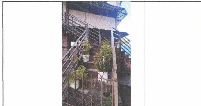
Foto 4: Lijado, cepillado y pintura de baranda de gradas que va hacia las aulas de segundo nivel 2 x5 ML, 10 ML
