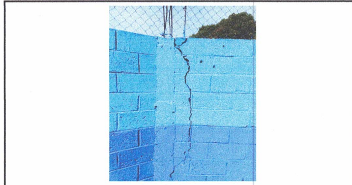
Foto 2: Mantenimiento de muro perimetral (Reforzamiento de 5 columnas de 4.00 mts lineales y vigas de 20x20 cms de grosor.)
