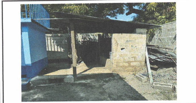
Foto 3: Sustitución de estructura de soporte de madera por metal y sustitución de lámina por lámina troquelada calibre 26
