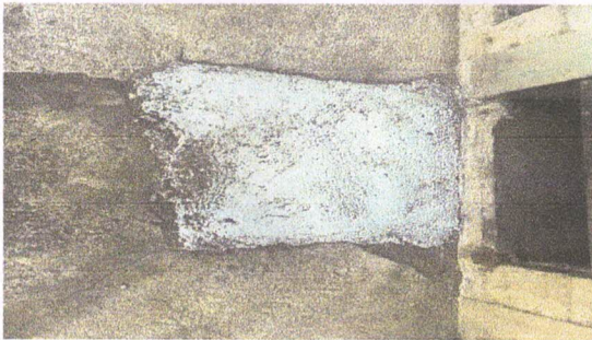
Foto 5: sustitucion de fosa septica
