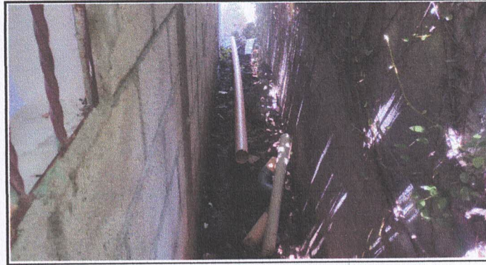
Foto 10: Módulo Red de Drenaje. Mantenimiento red de drenaje (reposición de tubería + reposición de concreto).
