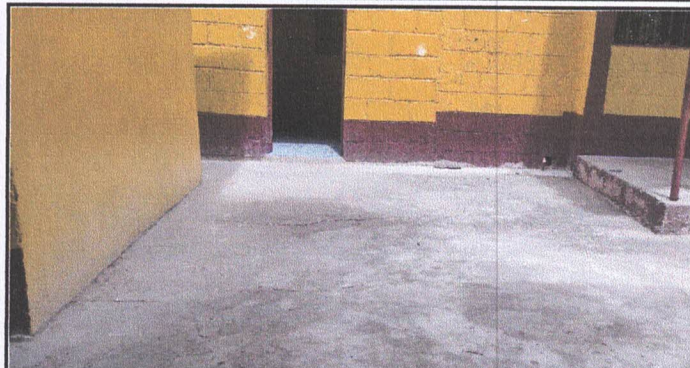
Foto 14: Módulo Losa de Patio. Demolición y retiro de piso de concreto existente en patio y sustitución de torta de piso de concreto en patio.
