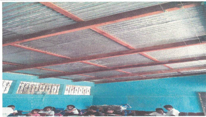
Cambio de madera por estructura metálica y lamina aluzinc troquelada calibre 26 en aulas
