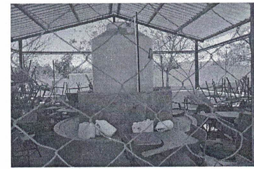
Foto 6: lavamanos circular que deberá ser reparado en su base, tuberías de instalación y llaves.
