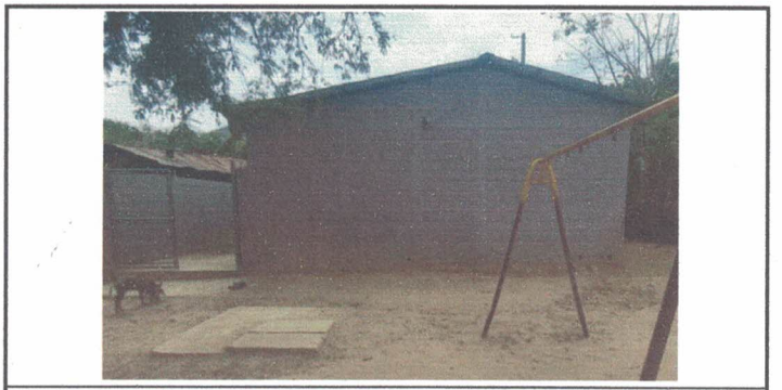
Foto 12: Dentro de este Renglón Especial, se considera la necesidad de Realizar una Limpieza a la Fosa Septica Existente y la Construcción de 1 Pozo de Absorción para que el Sistema de Tratamiento de Aguas Residuales quede funcionando correctamente.
