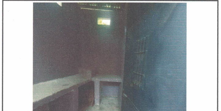
Foto 8: Se contempla la Instalación de 1 Estufa Rura con su Chimenea Metalica en Tubo Galvanizado Ø 3" con sus respectivos Accesorios.
