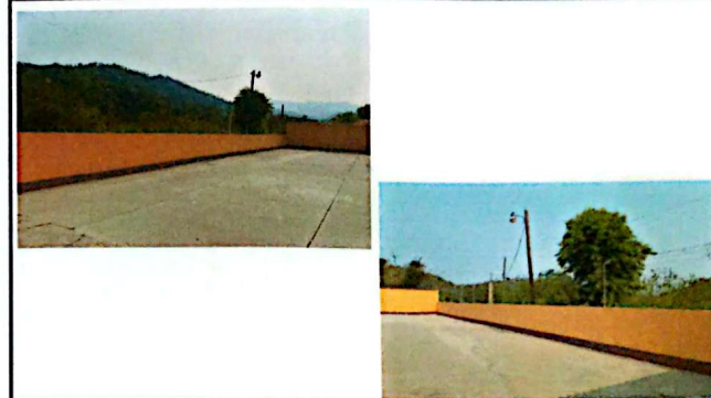
Foto 4: Levantamiento y aplicación de repello y cernido en pared, aplicación de pintura en muro, colocación de parte de agua de teja prefabricada.
