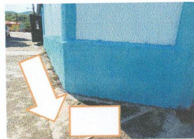
Foto 6: Instalación tubería PVC para aguas negras e instalación caja de registro
