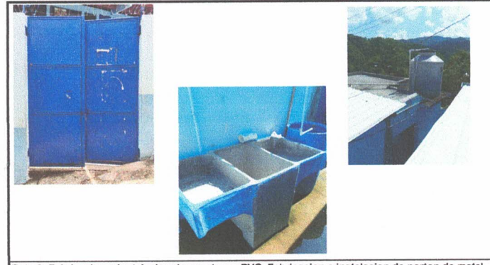
Foto 6: Fabricacion e instalacion de venetanas PVC, Fabricacion e instalacion de porton de metal de ingreso 2.00 X 2.15M, Instalacion de unidades luz (incluye interruptor, ducto, cable electrico, plafonera, bombillas), Instalacion de inodoro, Instalacion de tubo para agua potable y Instalacion de chorro.
