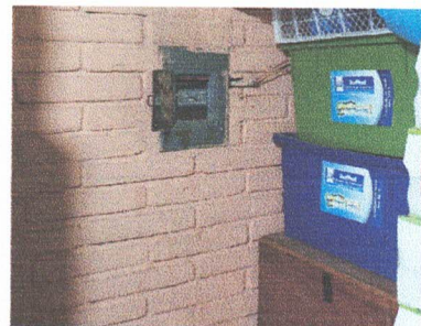
Foto 6: sustitución de caja y flipones
