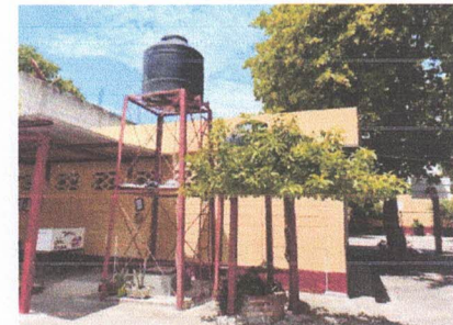
Foto 12: Sustitucion de depósito de agua de 2,500 litros
