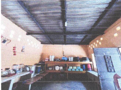
Foto7: Sustitución de focos ahorradores, plafoneras y tomacorrientes
