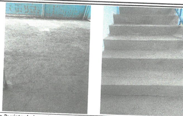
Foto 2: vista de losa de patio y gradas reparadas
