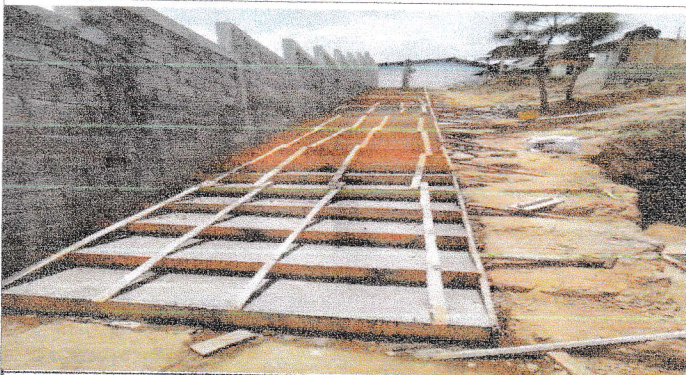
Foto 3: Fundición de gradas de concreto de 3 pulgadas de espesor
