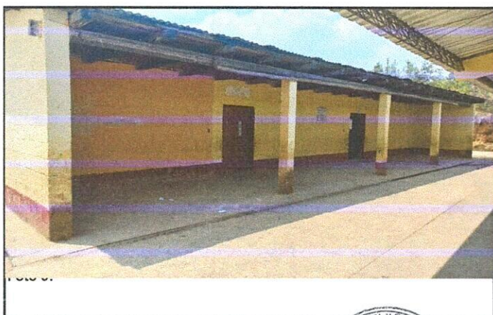
Foto3: Vista de la cubierta de techo, estas dos aulas se remozará con el cambio de techo
