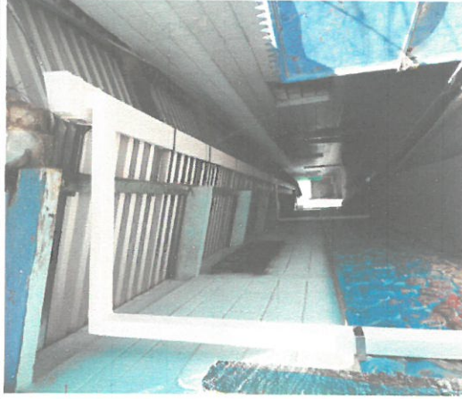
Foto 5: Sustitución de canal de metal por canal de PVC.
