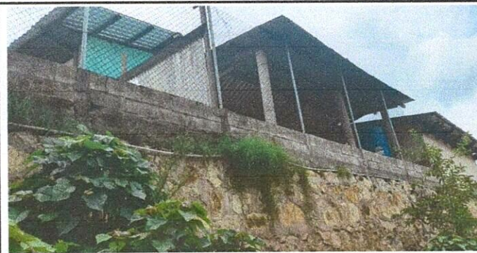
Foto 5: Reforzamiento del muro con columnas sapatas, cambio de malla por pared de blok con ventanas grandes sin vidrieras
