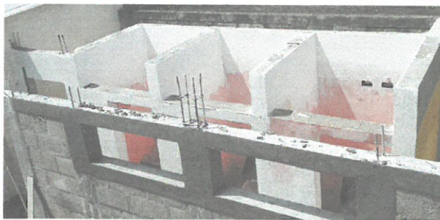
Elevación y nivelación de paredes de baños ya terminados.
