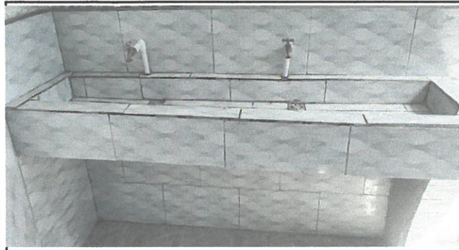
Foto 1: Baño de señoritas: instalación de azulejo en piso y paredes, lavamanos de concreto, reemplazo de inodoros, plomería completa.
